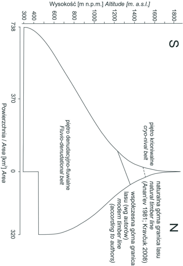
Ryc. 7. Wysokościowe zróżnicowanie intensywności procesów morfogenetycznych i piętra morfogenetyczne masywu Świdowca na tle krzywych hipsograficznych skłonu N i S masywu. Fig. 7. Vertical differences in the intensity of morphogenetic processes and morphogenetic belts in the Syrtovets massif against the background of the hypsographic curves of the N and S slope of the area.
